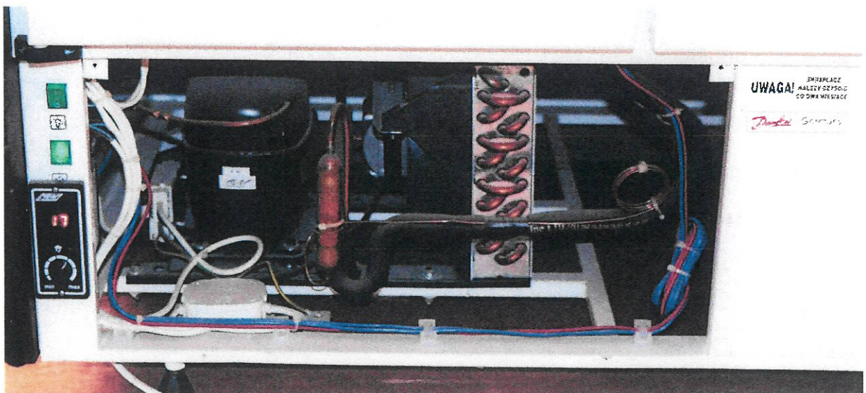
Obr. 9 (posuzovaná chlazená vitrína W12G, S/N: 30609692, chladičí agregát S.C. 10 CLX, R 507 - zjištěný stav ke dni 30. 04. 2024)
